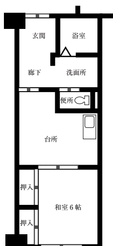
原田住宅 1DK
