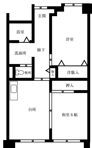
原田住宅 2DK
