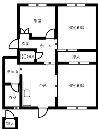
宮山住宅 3DK
