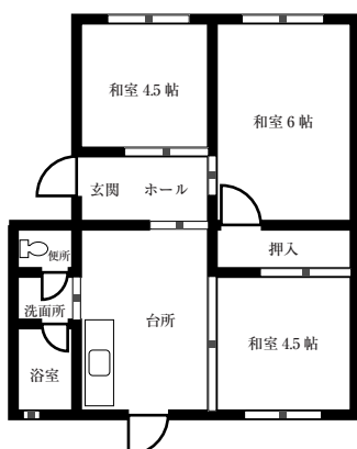
新千里南住宅 3DK
