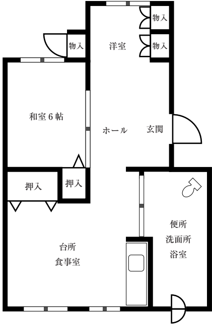
熊野住宅 2LDK(車いす常用障害者向)
